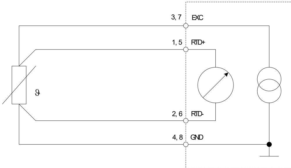
Abb. 4-4: Anschlussbeispiel: RTD-Sensoren (Vierleiterschaltung)
