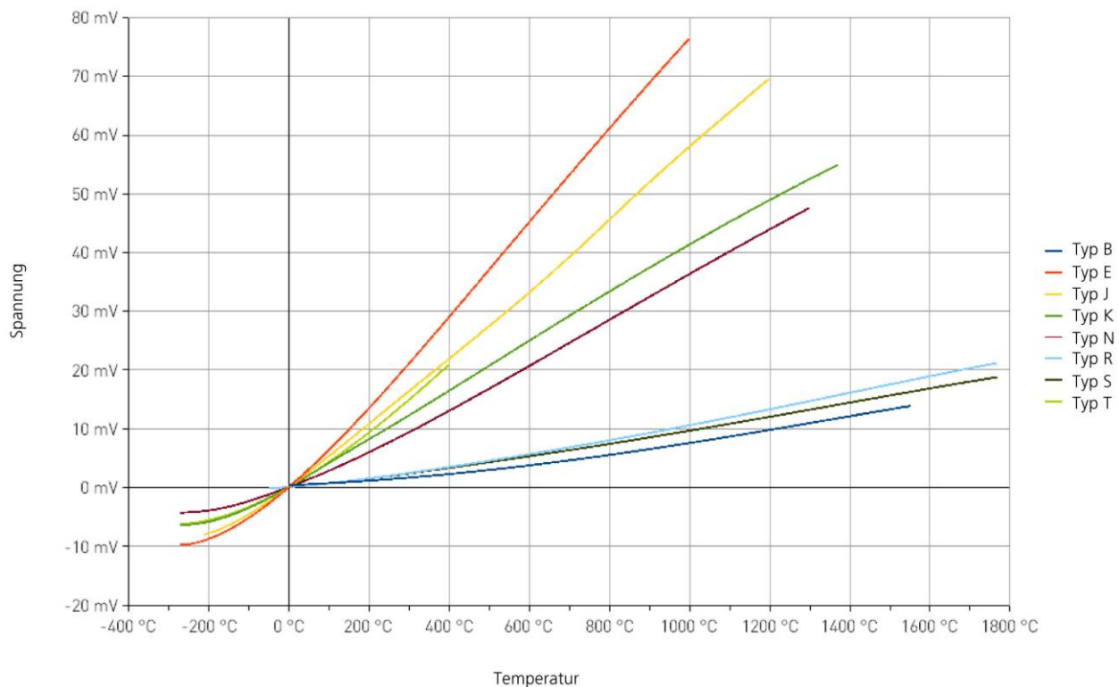
Abb. 3-2: Thermoelement-Typen: Auswahlkriterien
